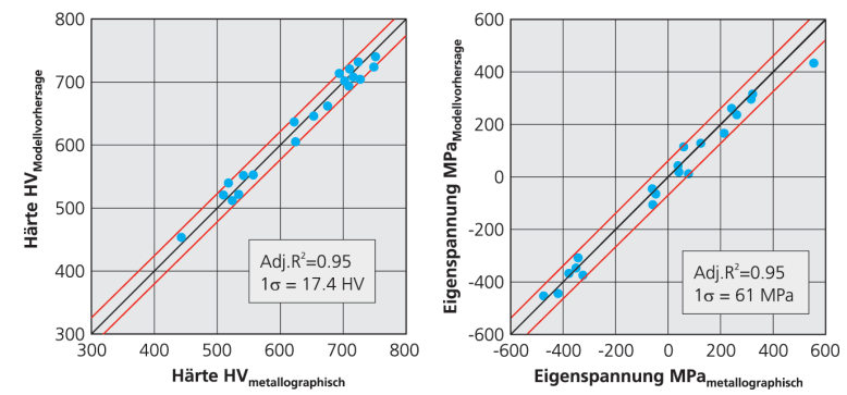
Links: Härteprüfung mit 3MA; Kalibrierung mit Diamant-Eindringhärte DPH 0.05 Rechts: Eigenspannungszustand mit 3MA gemessen; Kalibrierung mit Röntgen-Diffraktion
